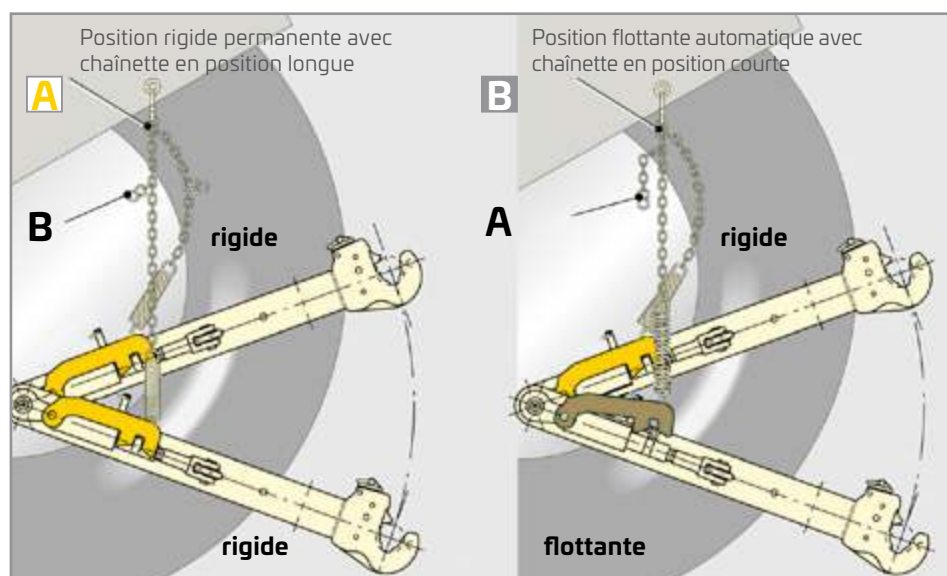
Position rigide
